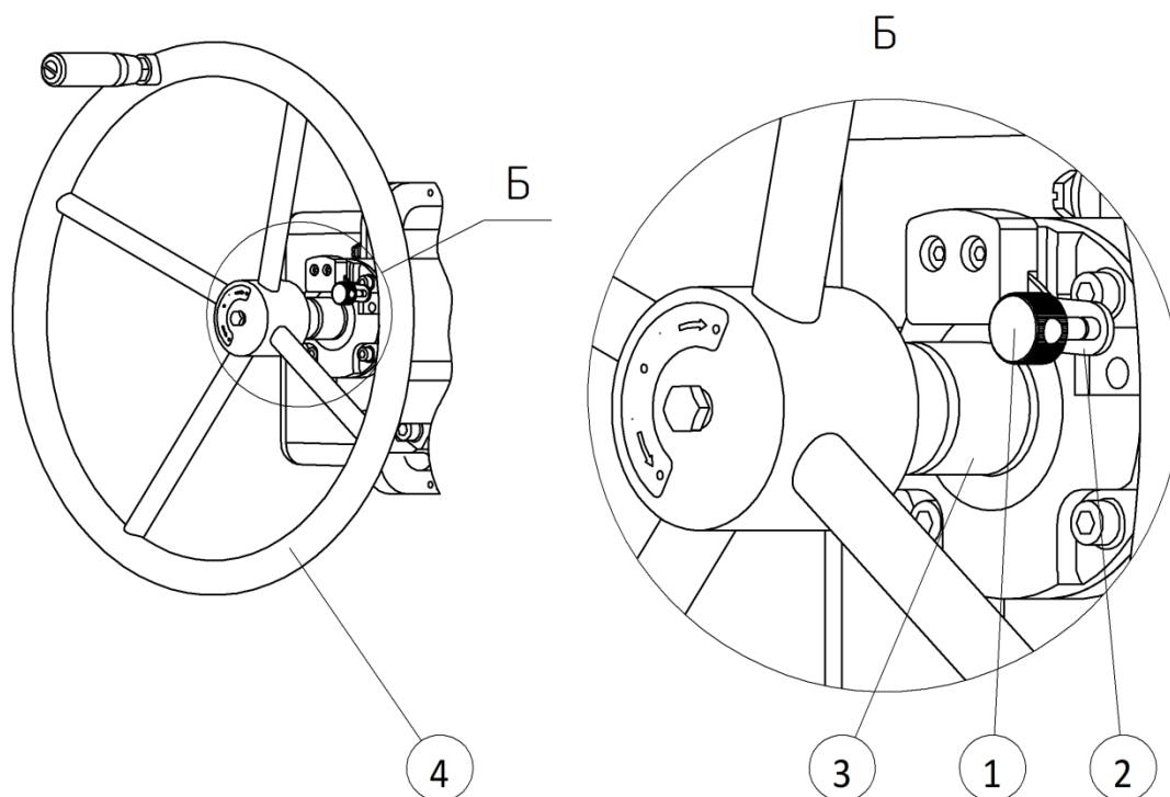
Рисунок 16 – Переключение на ручное управление
