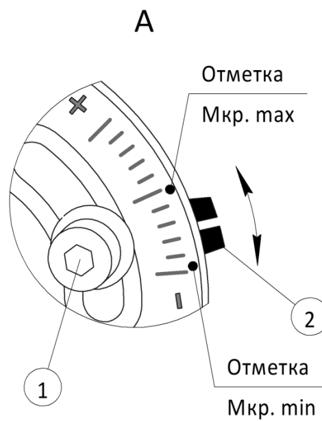
Рисунок 7 – Настройка момента выключения – закрытие.
