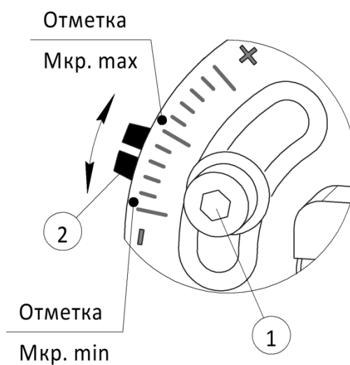
Рисунок 8 – Настройка момента выключения – открытие.
